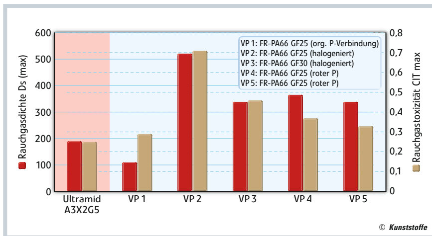
Bild 3. Emissionen im Brandfall: Vergleich von Polyamiden mit unterschiedlichem Flammenschutz, bezogen auf Rauchgasdichte Ds(max) (links) und Rauchgas-toxizität CIT max (rechts); (VP: Vergleichsprodukt) (Quelle: [8])
