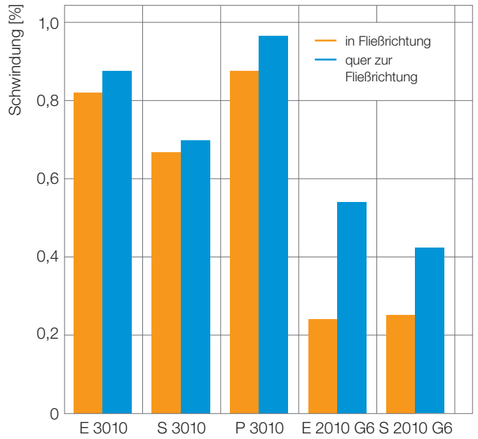
Abb. 43: Schwindungswerte verschiedener Ultrason®-Typen in und quer zur Fließrichtung
