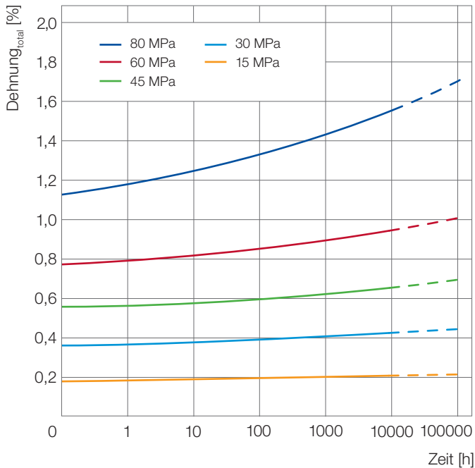
Abb. 16: Kriechkurven nach ISO 899 für Ultrason® S 2010 G6 bei 23 °C
