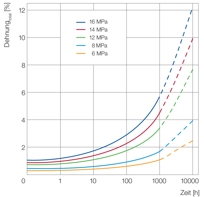
Abb. 15: Kriechkurven nach ISO 899 für Ultrason® P 3010 bei 180 °C
