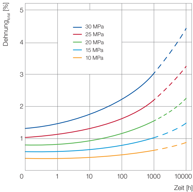
Abb. 13: Kriechkurven nach ISO 899 für Ultrason® E 3010 bei 140 °C
