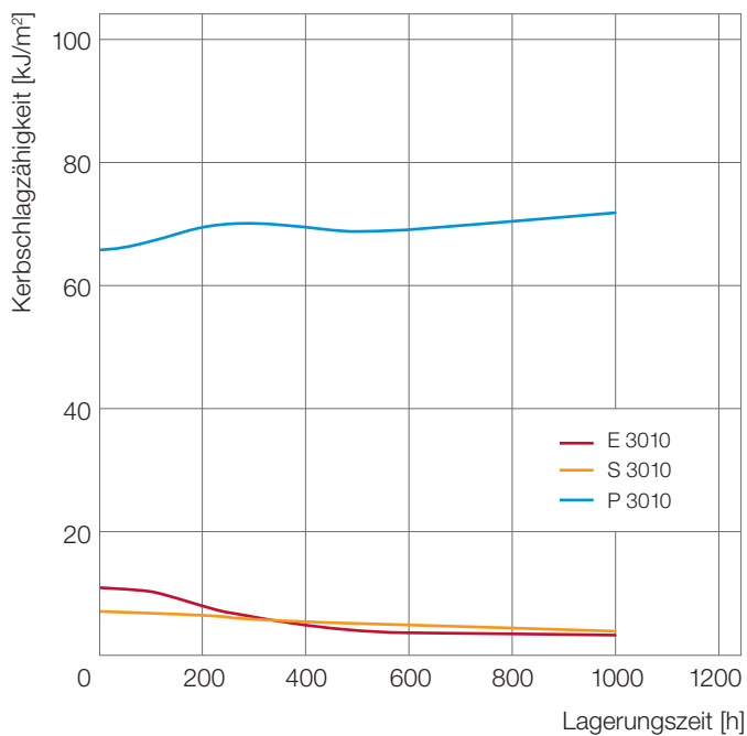
Abb. 35: Beständigkeit von Ultrason® gegen FAM B bei 23°C
