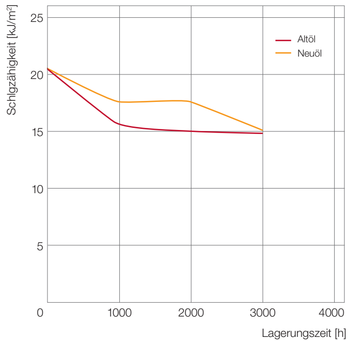
Abb. 33: Beständigkeit von Ultrason® KR 4113 gegen Motoröl Total 5W30 bei 150°C
