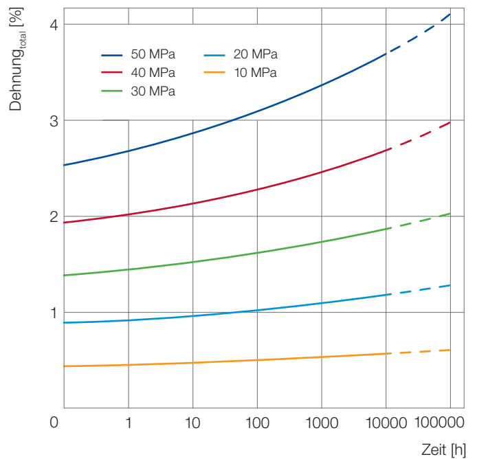
Abb. 11: Kriechkurven nach ISO 899 für Ultrason® E 3010 bei 23°C
