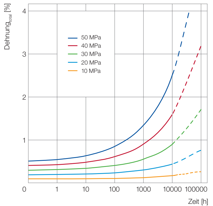
Abb. 20: Kriechkurven nach ISO 899 für Ultrason® E 2010 G6 bei 180°C
