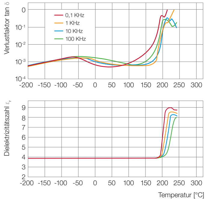
Abb. 39: Dielektrischer Verlustfaktor \tan \delta und Dielektrizitätszahl \epsilon_r von Ultrason® S 2010 in Abhängigkeit von der Temperatur
