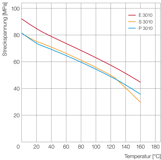
Abb. 4: Temperaturabhängigkeit der Streckspannung (trocken)
