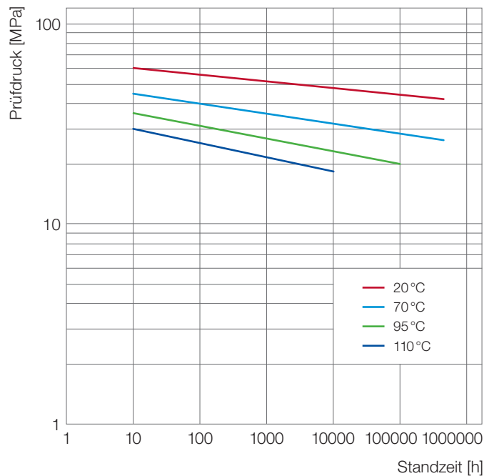
Abb. 27: Zeitstandinnendruck-Diagramm für Ultrason® P bei verschiedenen Temperaturen (ISO 9080)
