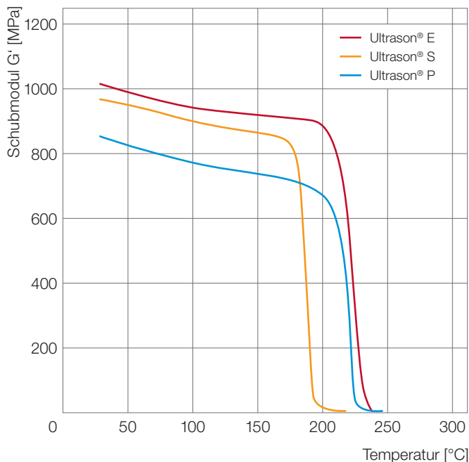
Abb. 1: Schubmodulkurven nach ISO 6721
