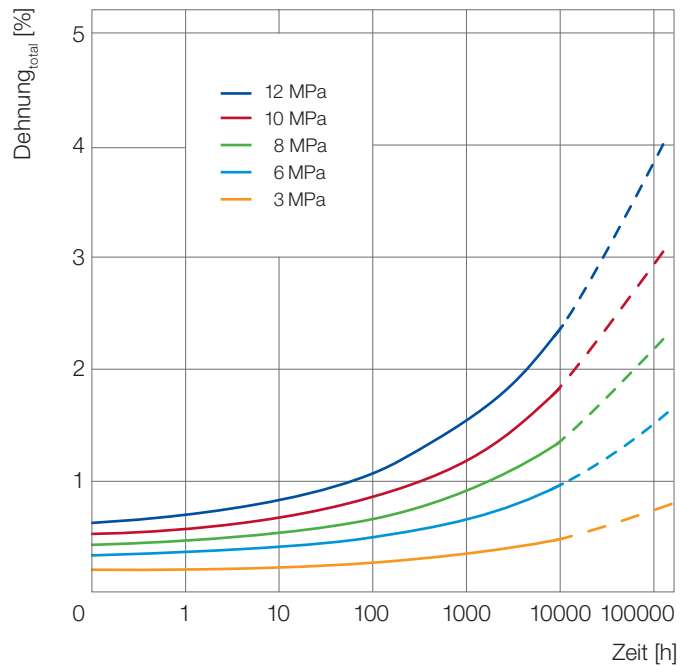
Abb. 14: Kriechkurven nach ISO 899 für Ultrason® E 3010 bei 180 °C
