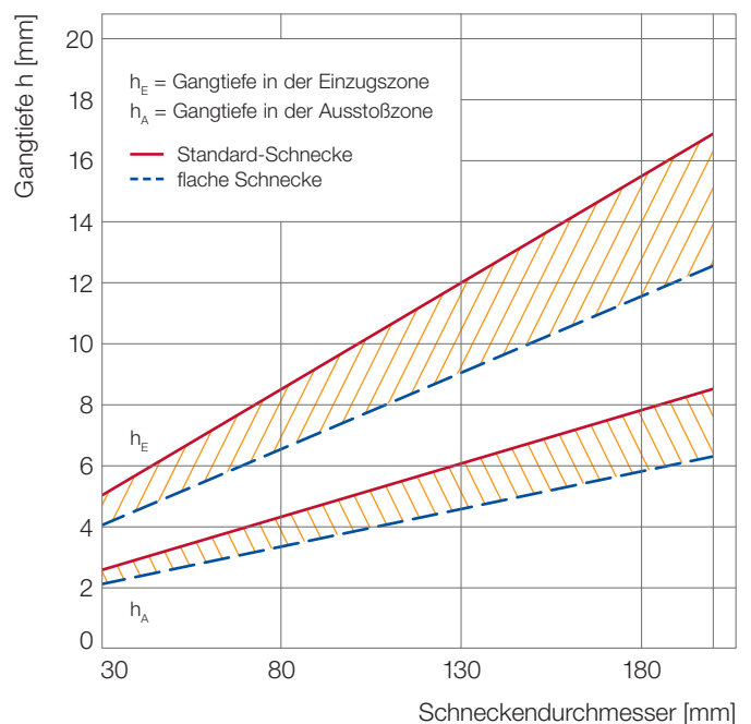
Abb. 42: Schneckengangtiefen von Dreizonenschnecken für Spritzgießmaschinen
