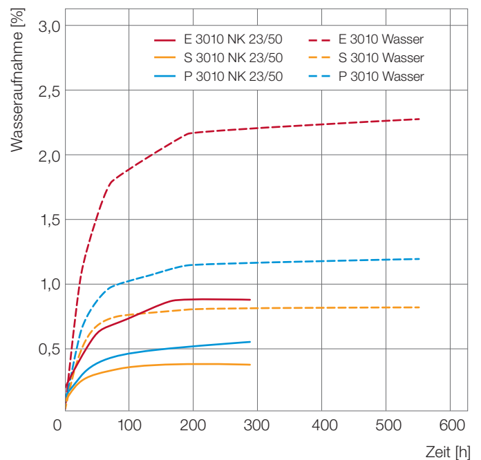
Abb. 41: Wasseraufnahme von Ultrason® in Abhängigkeit von der Lagerzeit (bei Normklima und getaucht), 2 mm Probekörperstärke
