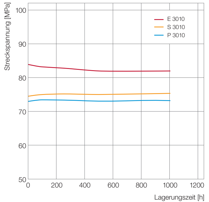
Abb. 36: Beständigkeit von Ultrason® gegen Glykol (50%-ig in Wasser) bei 23°C
