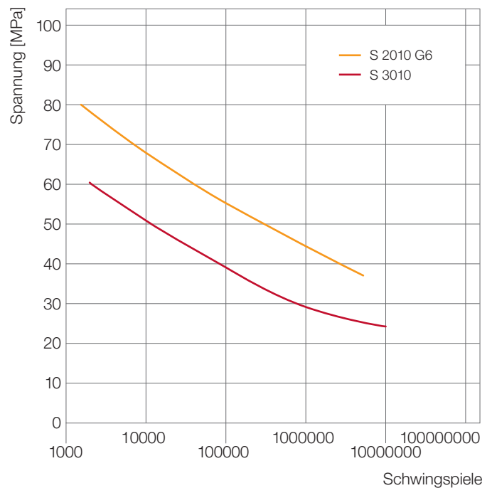
Abb. 22: Wöhlerdiagramm Ultrason® S 3010 und S 2010 G6 bei 23°C
