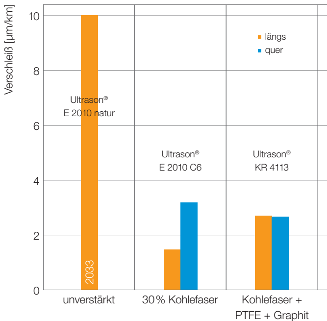
Abb. 23: Verschleißverhalten Tribosystem: Stift-Scheibenapparatur, Flächenpressung p = 1 \text{ MPa} , Grundkörper Aluminium mit 6,7 \text{ µm} Rauheit (trocken)
