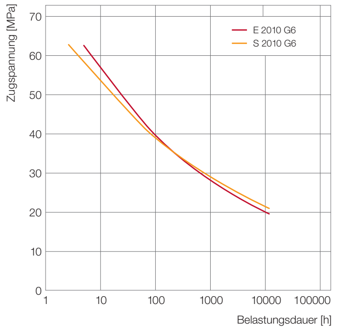
Abb. 26: Zeitstandfestigkeit von Ultrason® in Wasser bei 95°C
