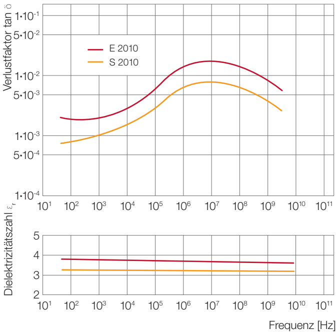
Abb. 38: Dielektrischer Verlustfaktor \tan \delta und Dielektrizitätszahl \epsilon_r von Ultrason® S 2010 und E 2010 in Abhängigkeit von der Frequenz (bei Normklima)
