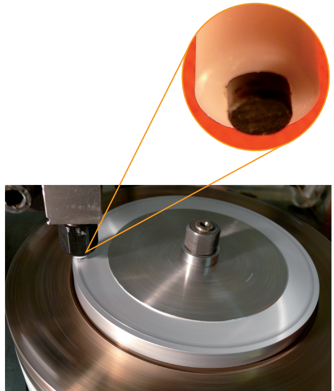
Abb. 23: Verschleißverhalten Tribosystem: Stift-Scheibenapparatur, Flächenpressung p = 1 \text{ MPa} , Grundkörper Aluminium mit 6,7 \text{ µm} Rauheit (trocken)
