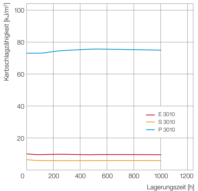
Abb. 37: Beständigkeit von Ultrason® gegen Glykol (50%-ig in Wasser) bei 23°C
