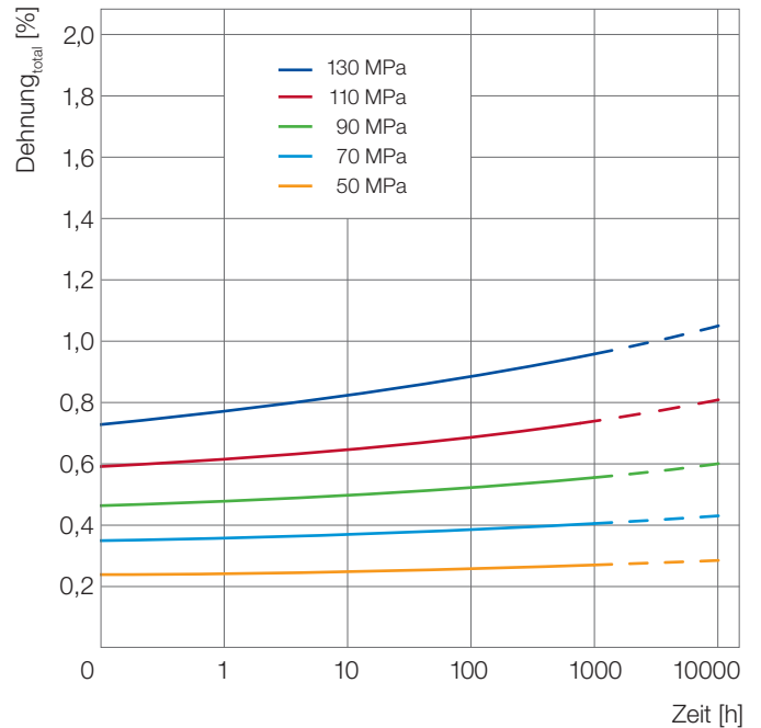
Abb. 18: Kriechkurven nach ISO 899 für Ultrason® E 2010 C6 bei 23 °C
