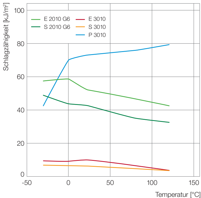
Abb. 8: Schlagzähigkeit in Abhängigkeit von der Temperatur (ungekerbt nach ISO 179/1eU) bei glasfaserverstärkten und gekerbt nach ISO 179/1eA bei unverstärkten Typen)
