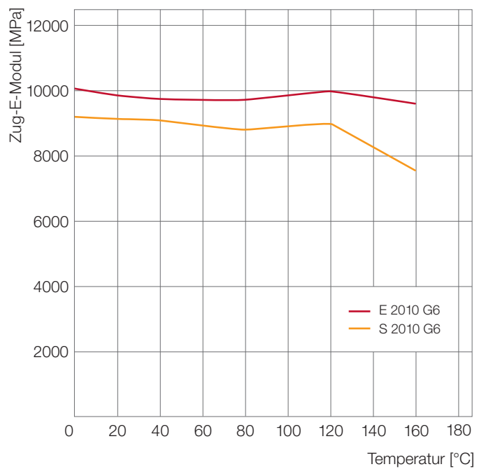
Abb. 7: Elastizitätsmodul (nach ISO 527) in Abhängigkeit von der Temperatur (trocken)
