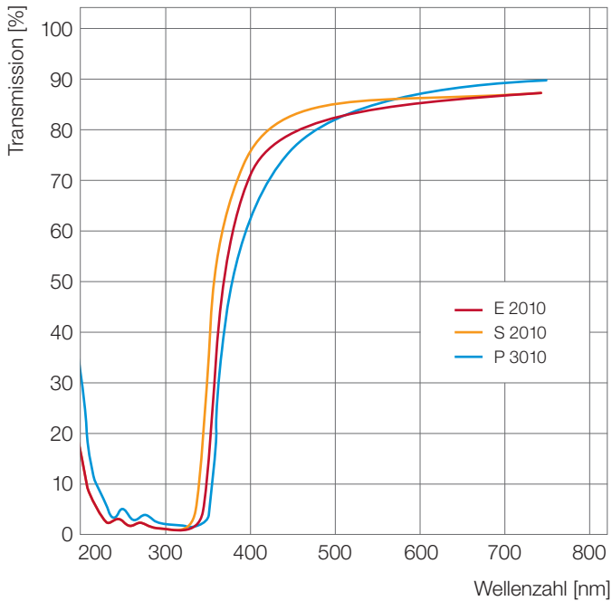
Abb. 30: Transmissionseigenschaften von Ultrason® (2 mm Plättchen)
