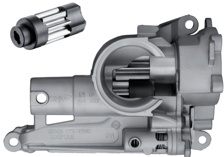
Ölpumpe mit Ölregelkolben
