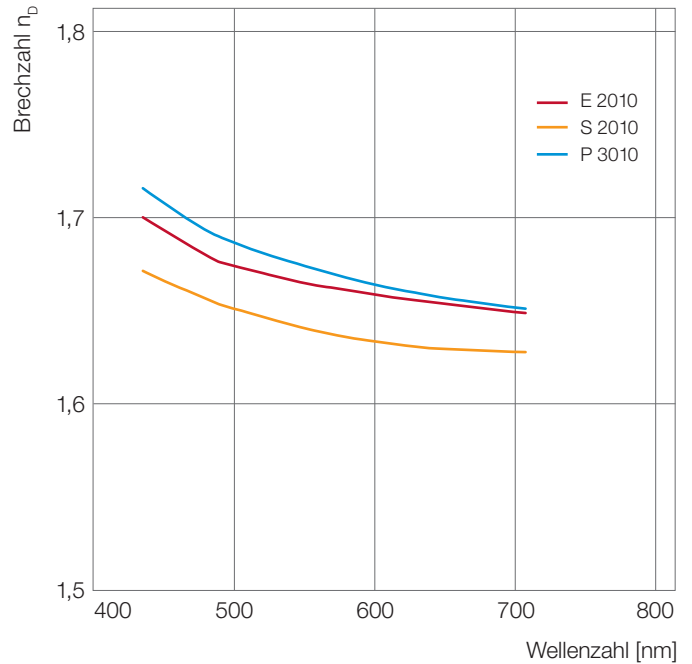
Abb. 31: Brechzahl von Ultrason® in Abhängigkeit von der Wellenlänge (2 mm Plättchen)
