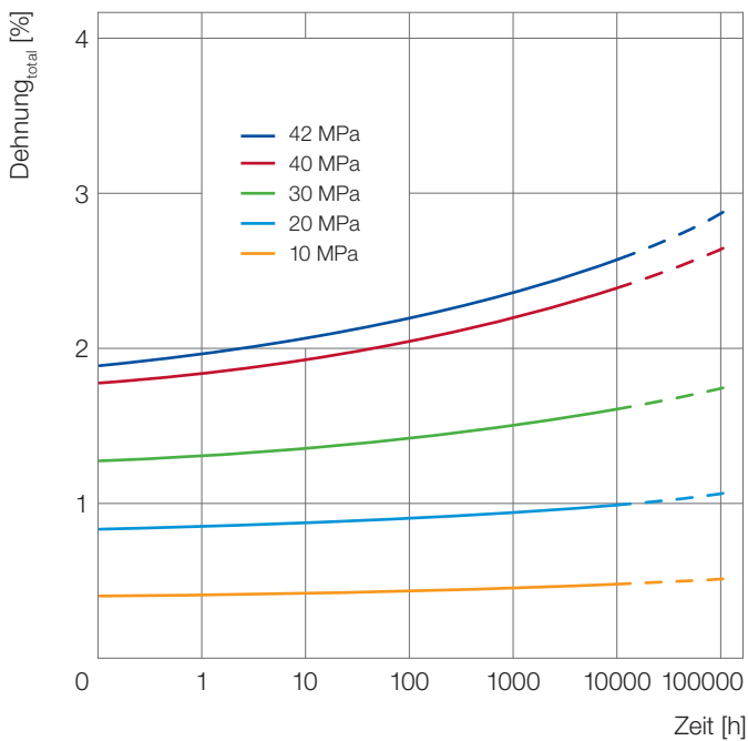
Abb. 10: Kriechkurven nach ISO 899 für Ultrason® S 3010 bei 23°C
