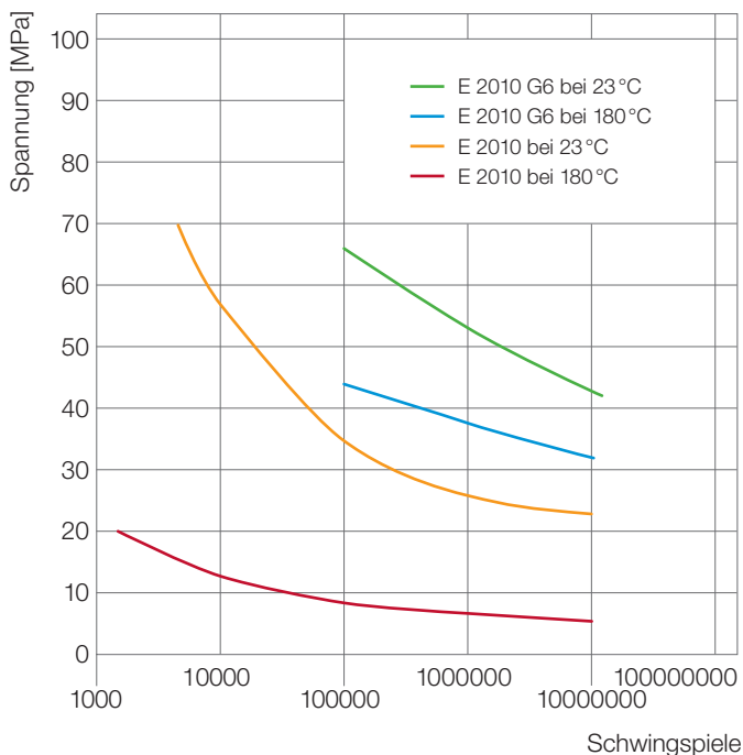
Abb. 21: Wöhlerdiagramm Ultrason® E 2010 und E 2010 G6 bei 23°C und 180°C
