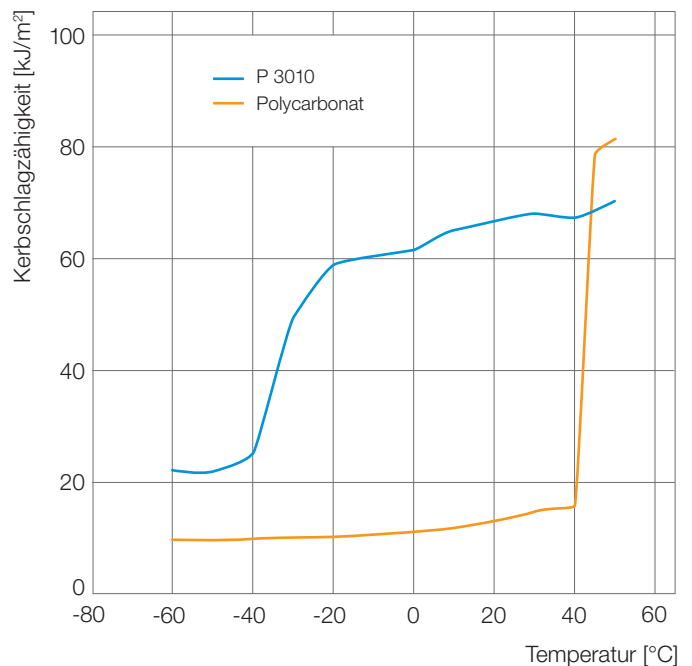
Abb. 9: Kerbschlagzähigkeit in Abhängigkeit von der Temperatur (ISO 179/1eA); Vergleich Ultrason® P mit einem Standard-Polycarbonat
