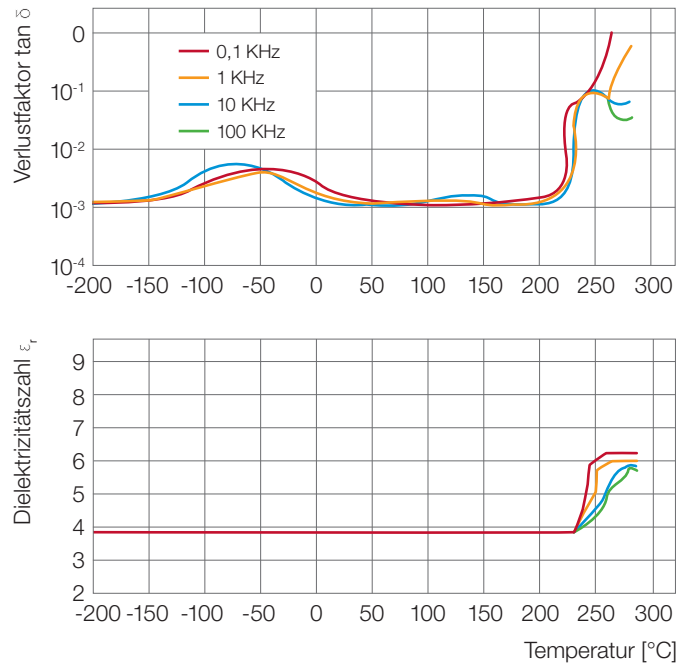
Abb. 40: Dielektrischer Verlustfaktor \tan \delta und Dielektrizitätszahl \epsilon_r von Ultrason® E 2010 in Abhängigkeit von der Temperatur
