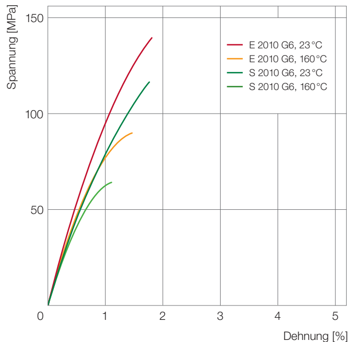
Abb. 3: Spannungs-Dehnungsdiagramme nach ISO 527 bis zur Reißgrenze, bei RT und 160°C
