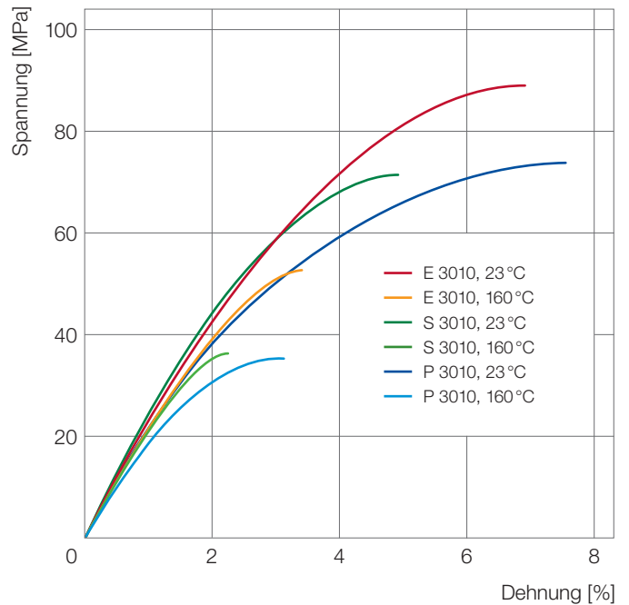
Abb. 2: Spannungs-Dehnungsdiagramme nach ISO 527 bis zur Streckgrenze, bei RT und 160°C
