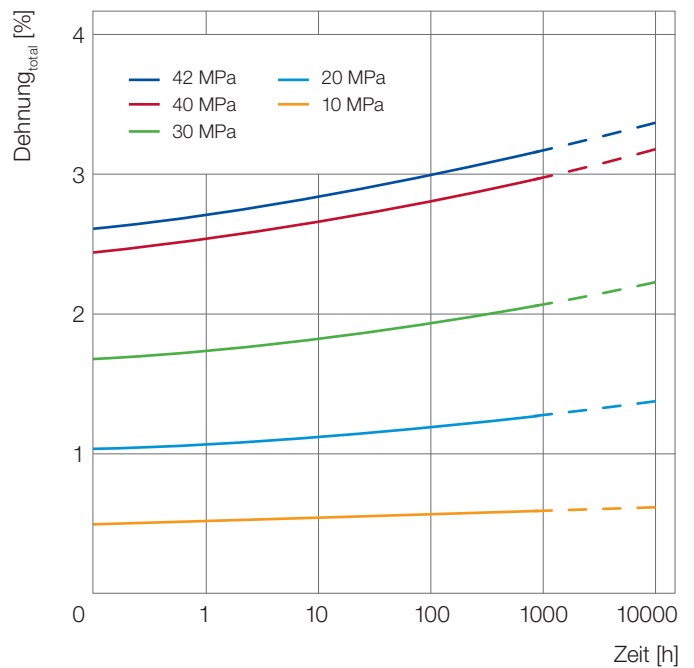
Abb. 12: Kriechkurven nach ISO 899 für Ultrason® P 3010 bei 23°C
