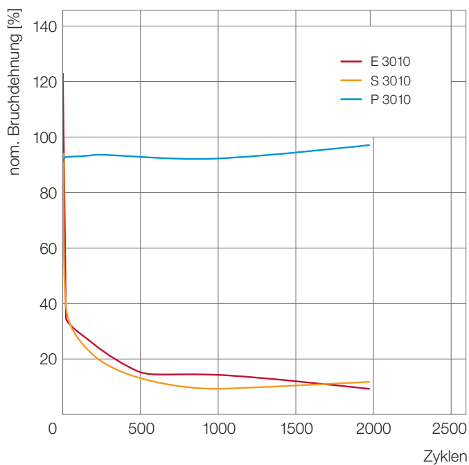
Abb. 29: Heißdampfsterilisation von Ultrason® bei 134 °C
