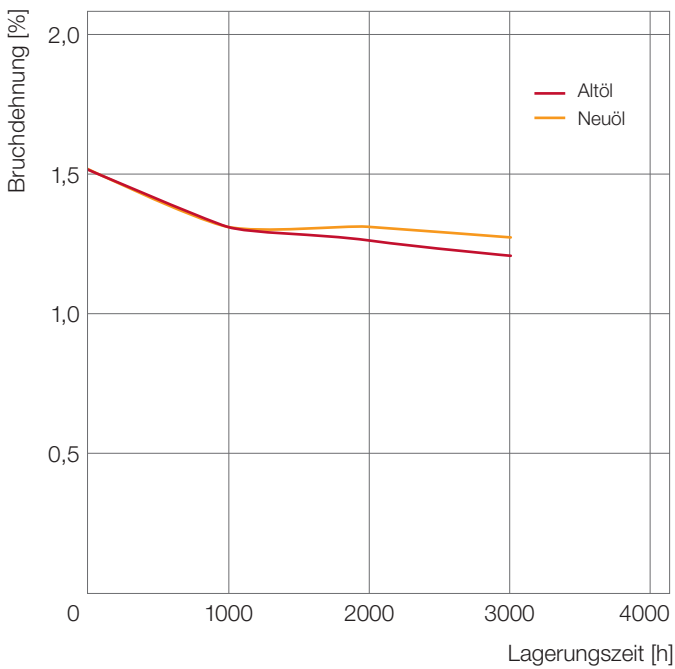
Abb. 32: Beständigkeit von Ultrason® KR 4113 gegen Motoröl Total 5W30 bei 150°C
