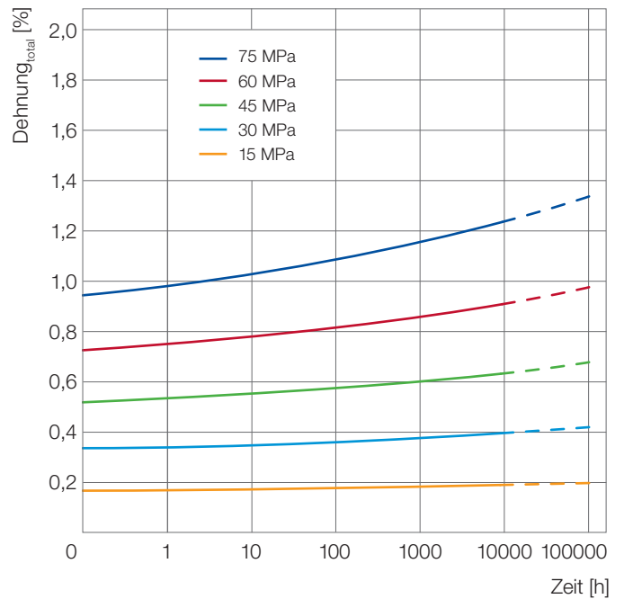
Abb. 17: Kriechkurven nach ISO 899 für Ultrason® E 2010 G6 bei 23 °C
