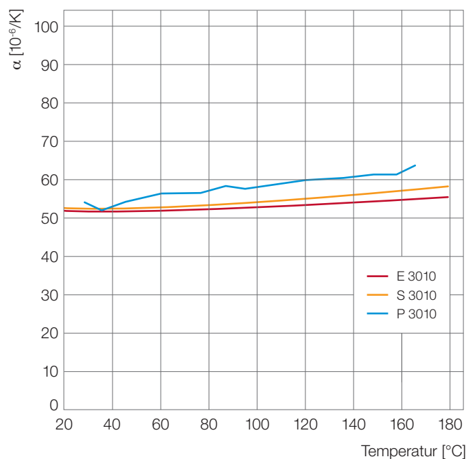
Abb. 24: Längenausdehnungskoeffizient nach DIN 53752
