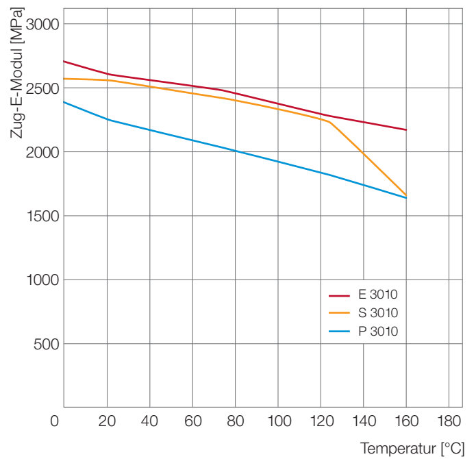
Abb. 6: Elastizitätsmodul (nach ISO 527) in Abhängigkeit von der Temperatur (trocken)
