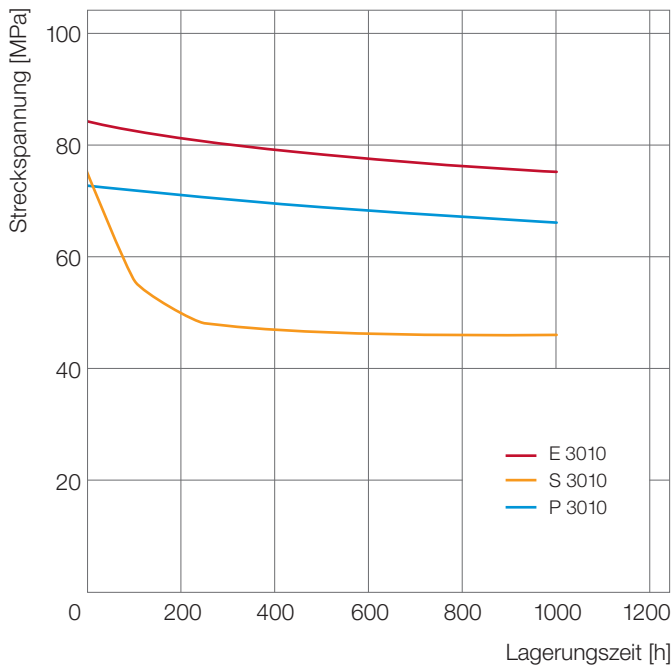
Abb. 34: Beständigkeit von Ultrason® gegen FAM B bei 23°C
