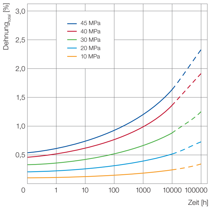
Abb. 19: Kriechkurven nach ISO 899 für Ultrason® S 2010 G6 bei 140°C
