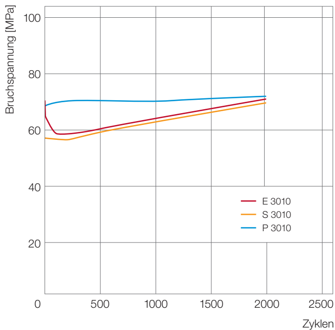
Abb. 28: Heißdampfsterilisation von Ultrason® bei 134 °C
