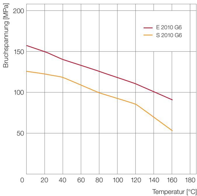
Abb. 5: Temperaturabhängigkeit der Bruchspannung (trocken)
