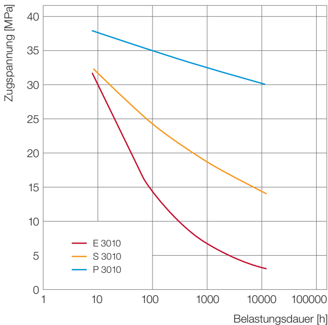
Abb. 25: Zeitstandfestigkeit von Ultrason® in Wasser bei 95°C
