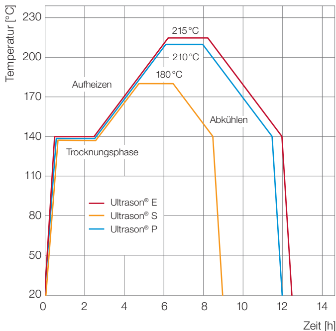
Abb. 44: Tempern von Ultrason®
